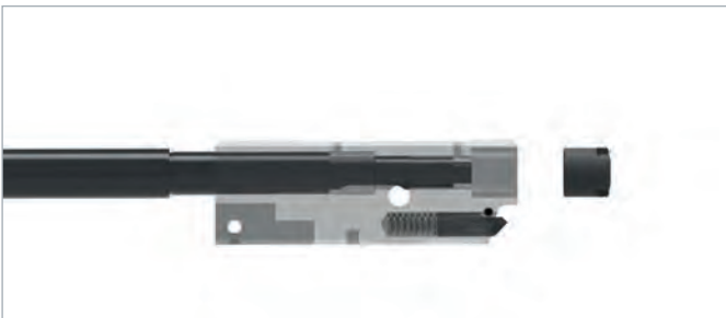
Wechselbarer Lauf mit 1/2" UNF Mündungsgewinde Changeable barrel with 1/2" UNF muzzle thread
